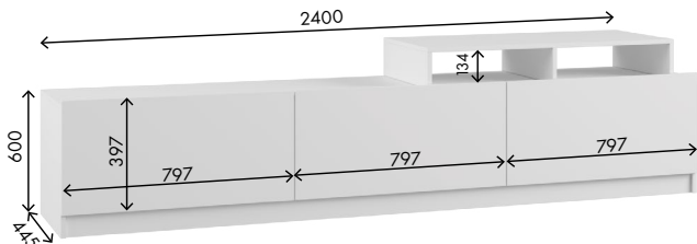
Гостиная ТМ (тумба) Габариты ДхВхГ, мм: 2400х600х445
