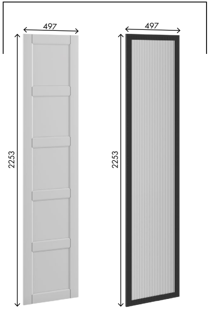
Фасад 50 см Габариты ДхВ, мм: 497х2253
