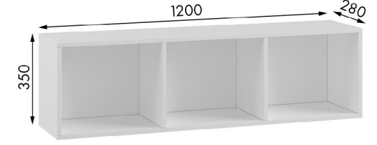
Полка большая Габариты ДхВхГ, мм: 1200x350x280
