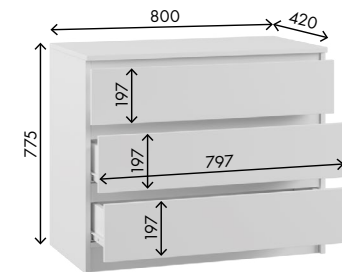
Комод К3М Габариты ДхВхГ, мм: 800x775x420
