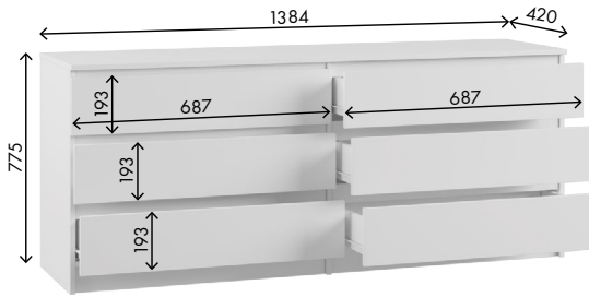
Комод 1384 Габариты ДхВхГ, мм: 1384x775x420
