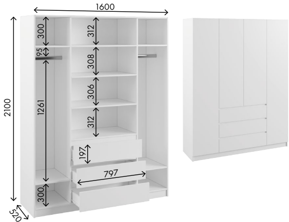
Шкаф 4-х створчатый Габариты ДхВхГ, мм: 1600х2100х520
