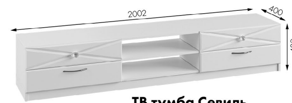
ТВ тумба Севиль Габариты ДхВхГ, мм: 2002х480х400
