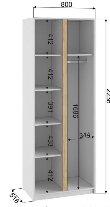
Шкаф Фаворит 800-02 Габариты ДхВхГ, мм: 800х2236х516
