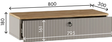
Подвесная консоль Габариты ДхВхГ, мм: 800х180х300
