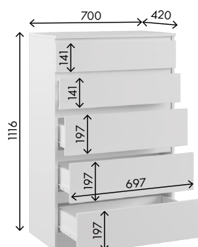
Комод К700 Габариты ДхВхГ, мм: 700x1116x420
