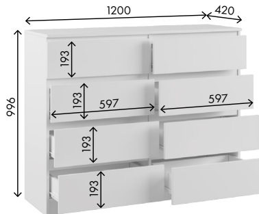
Комод 1200.8 Габариты ДхВхГ, мм: 1200x996x420
