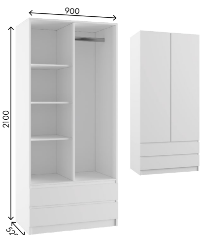
Шкаф ШМ Габариты ДхВхГ, мм: 900х2100х520
