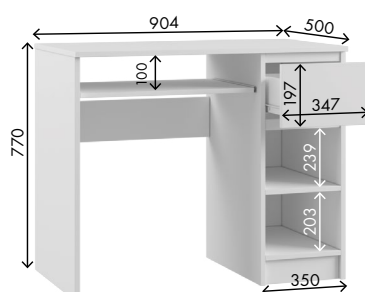
Стол письменный СМП1Д Габариты ДхВхГ, мм: 904х770х500
