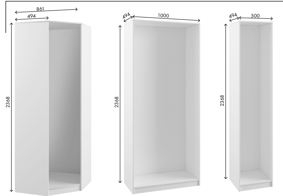
Каркас угловой Габариты ДхВхГ, мм: 861х2368х861
