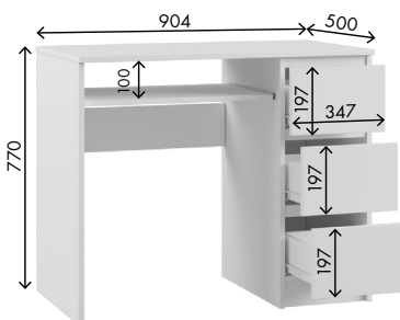
Стол письменный СМП900 Габариты ДхВхГ, мм: 904х770х500
