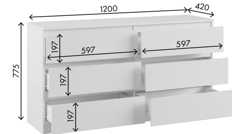
Комод К6М Габариты ДхВхГ, мм: 1200x775x420
