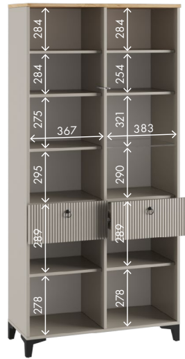
Шкаф 2-х створчатый Габариты ДхВхГ, мм: 900х2100х500
