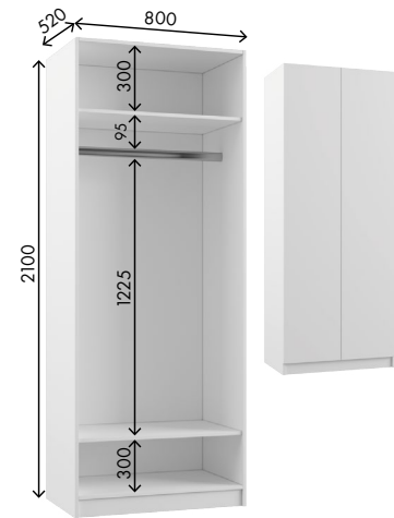
Шкаф ШМ2 Габариты ДхВхГ, мм: 800х2100х520
