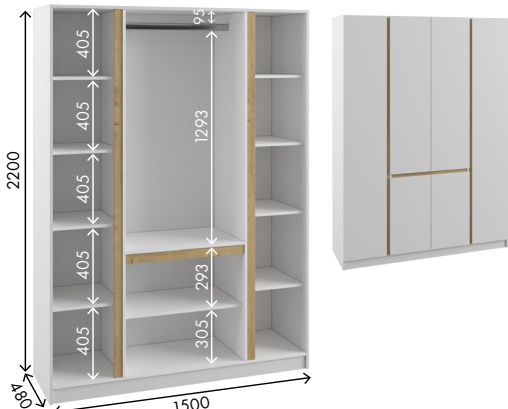
Шкаф М1500.4 Габариты ДхВхГ, мм: 1500х2200х480
