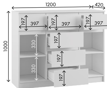
Комби 2 Габариты ДхВхГ, мм: 1200х1000х420
