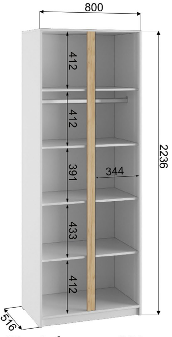
Шкаф Фаворит 800 Габариты ДхВхГ, мм: 800х2236х516
