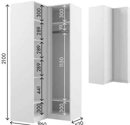
Шкаф ШМУ Габариты ДхВхГ, мм: (960х960)х2100х520
