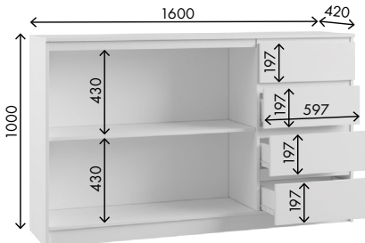
Комби 1 Габариты ДхВхГ, мм: 1600х1000х420
