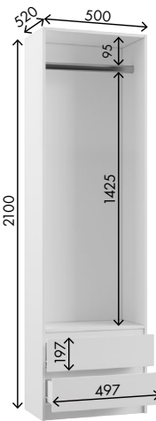
Пенал 3ПМ Габариты ДхВхГ, мм: 500х2100х520
