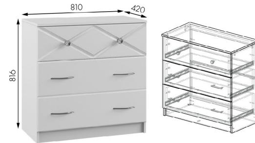
Комод 3 ящика Севиль Габариты ДхВхГ, мм: 810х816х420
