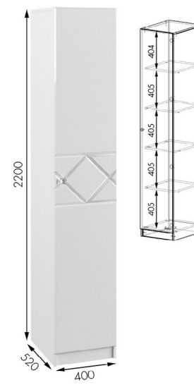
Пенал Севиль Габариты ДхВхГ, мм: 400х2200х520
