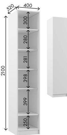
Пенал ДМ Габариты ДхВхГ, мм: 400х2100х520
