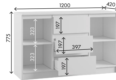
Тумба ТД3 Габариты ДхВхГ, мм: 1200х775х420
