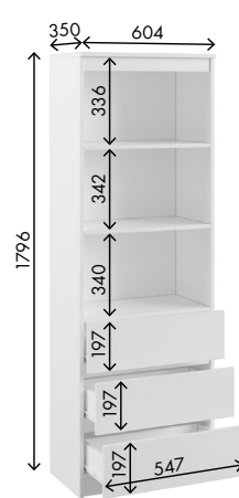
Стеллаж М600 Габариты ДхВхГ, мм: 600х1800х350
