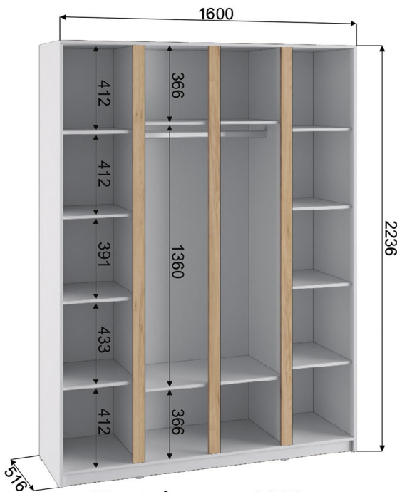
Шкаф Фаворит 1600 Габариты ДхВхГ, мм: 1600х2236х516
