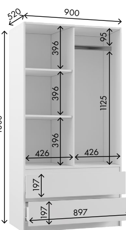
Шкаф Ш1800 Габариты ДхВхГ, мм: 900х1800х520
