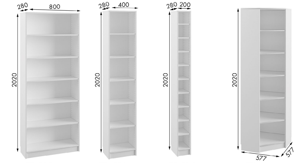
СБ-800 Габариты ДхВхГ, мм: 800x2020x280
