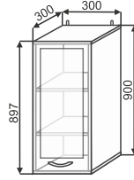
ШВС(2) 300 300x900x300
