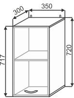
ШВ 350 350x720x300
