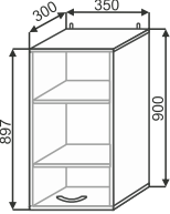
ШВ(2) 350 350x900x300
