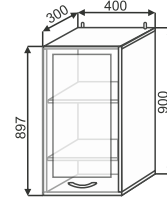
ШВС(2) 400 400x900x300
