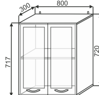
ШВС 800 800x720x300
