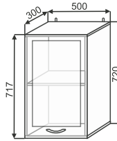
ШВС 500 500x720x300
