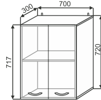
ШВ 700 700x720x300
