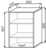
ШВ(2) 601 600x900x300
