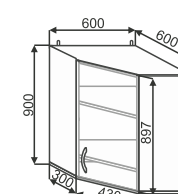
ШВУ(2) 600X600 600x900x600
