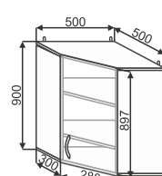
ШВУ(2) 500X500 500x900x500
