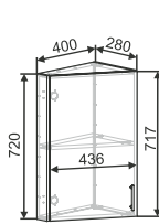
ШВУД 400 400x720x300
