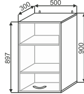
ШВ(2) 500 500x900x300
