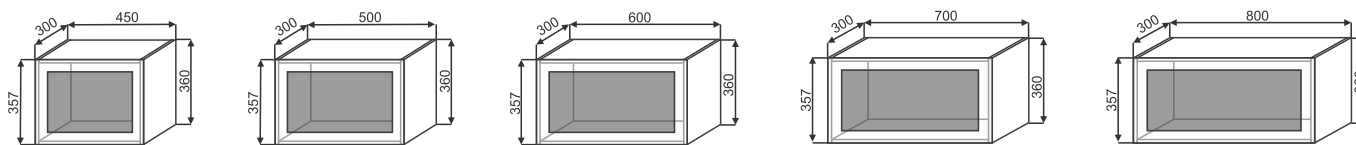
ВГС 450 450x360x300 ВГС 500 500x360x300 ВГС 600 600x360x300 ВГС 700 700x360x300 ВГС 800 800x360x300
