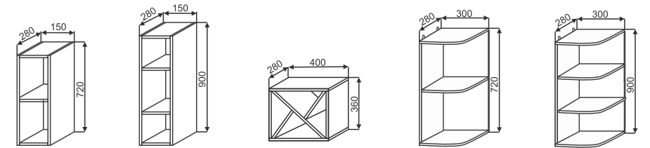
ПВ 150 150x720x280 ПВ(2) 150 150x900x280 ВБ 400 400x360x280 ШВПУ 300 300x720x280 ШВПУ(2) 300 300x900x280
