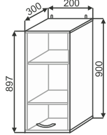
ШВ(2) 200 200x900x300
