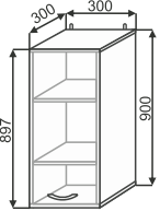
ШВ(2) 300 300x900x300
