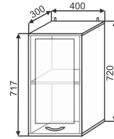
ШВС 400 400x720x300
