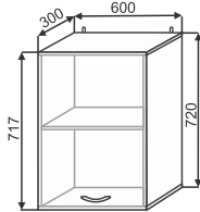
ШВ 601 600x720x300
