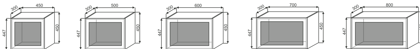
ВГС(2) 450 450x450x300 ВГС(2) 500 500x450x300 ВГС(2) 600 600x450x300 ВГС(2) 700 700x450x300 ВГС(2) 800 800x450x300
