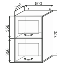
ШВБС 500 500x720x300
