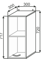
ШВ 300 300x720x300
