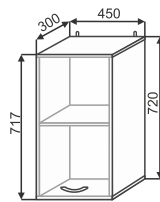
ШВ 450 450x720x300
