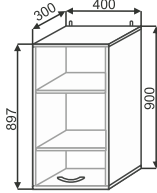
ШВ(2) 400 400x900x300
