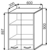
ШВ(2) 600 600x900x300
