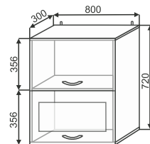
ШВБС(1) 800 800x720x300
