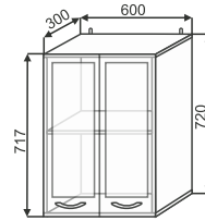
ШВС 600 600x720x300
