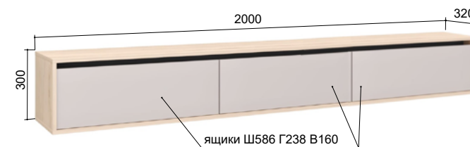
«Рэя» Тумба навесная 2000 мм 2000*320*300 мм
