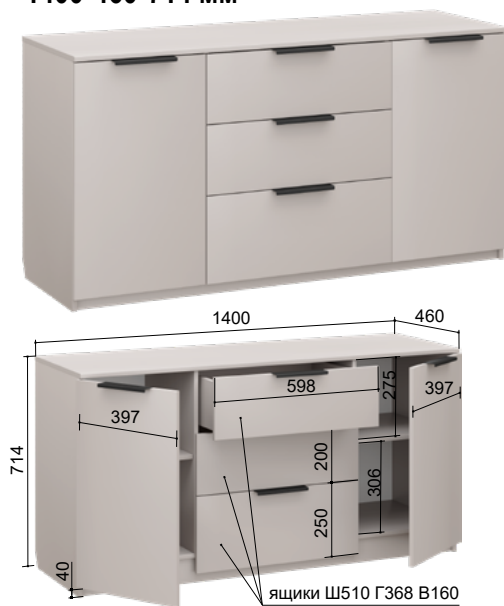
«Чарли» 9.1 Комод 1400*460*714 мм
