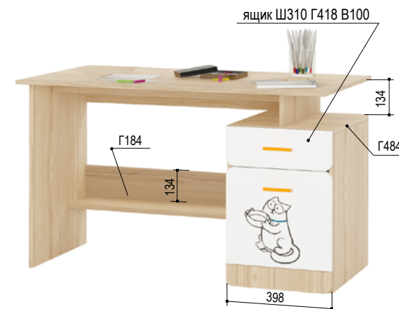
«Кот» 17 Письменный стол 1200*650*750 мм
