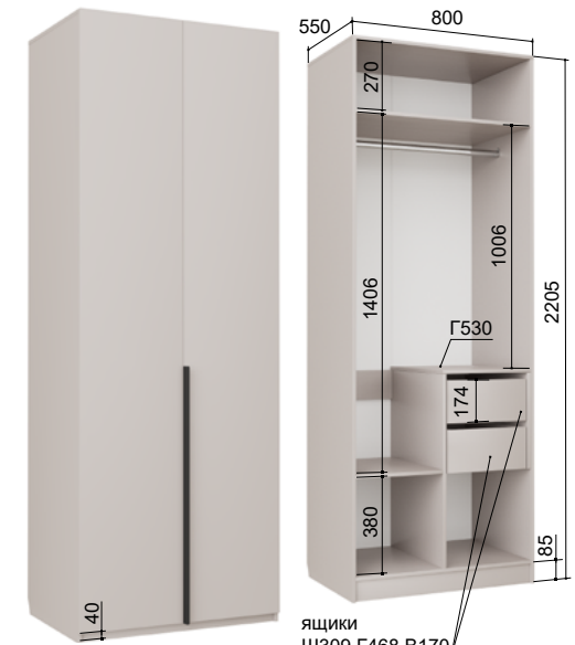
«Чарли» 22 Шкаф 2-створчатый 800*550*2205 мм
